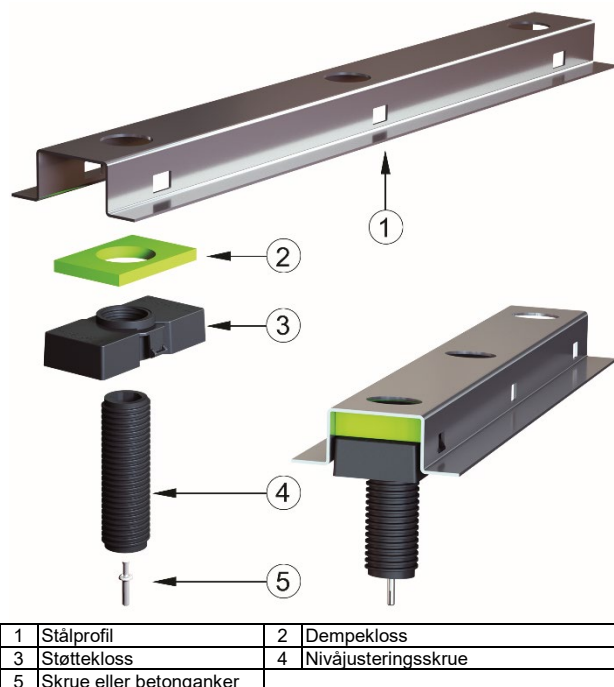
Fig. 1 Granab tilfarersystem, versjon 3000N12 (12 mm dempelement). Figuren viser de ulike komponentene oppdelt og sammensatt. Det er samme prinsipp for versjon 7000N og 9000N, men stålprofil og dempelementer varierer.
