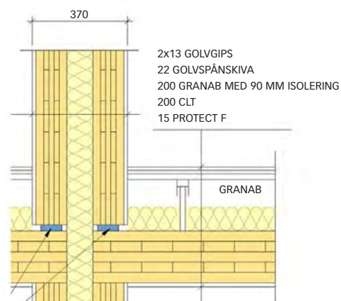
Exempel på lösning för att klara ljudkraven på massivträ.
